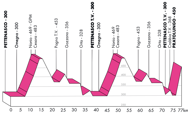
Altimetria complessiva
