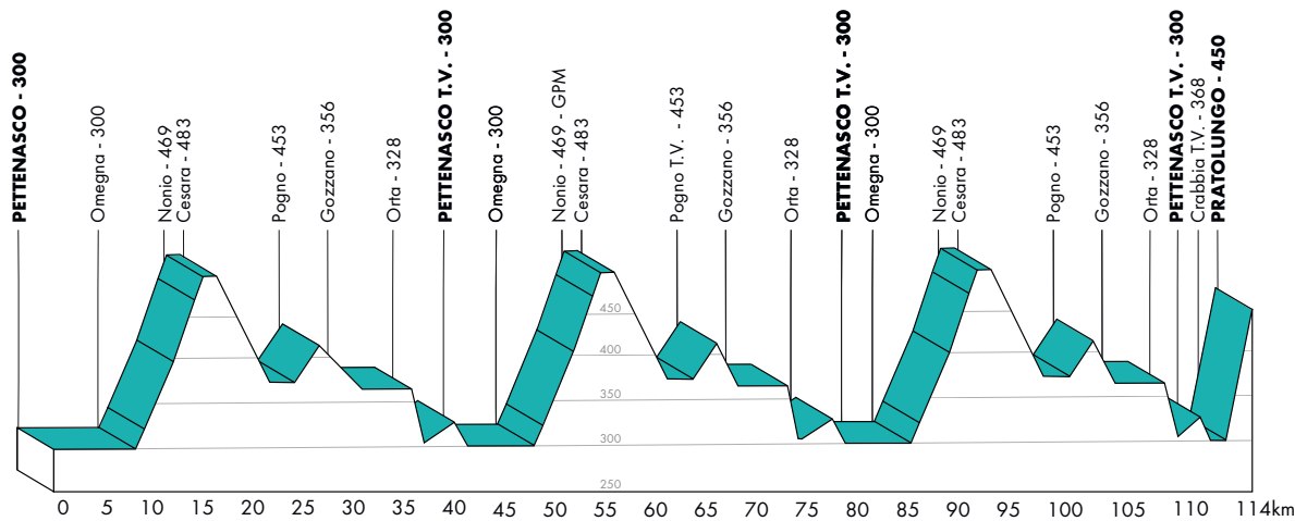
Altimetria complessiva
